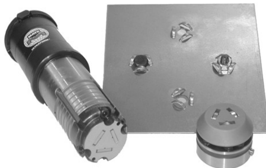
Obr. 1: Nástroj HexLock™ vyrábí spolehlivé a bezpečné uchycení pro šestihranné spojovací prvky v plechu
